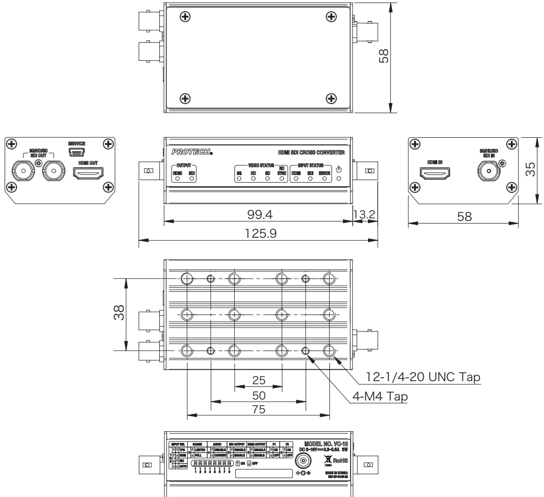
Outside dimension (unit: mm) 外形寸法図(単位:ミリ)
